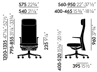
Pacific Chair avec dossier rembourré haut et accoudoirs fixes
