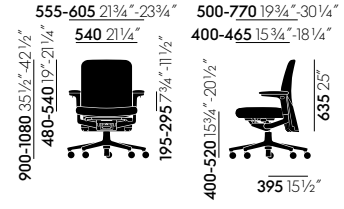
Pacific Chair avec dossier rembourré bas et accoudoirs 3D
