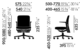
Pacific Chair avec dossier rembourré bas et accoudoirs fixes
