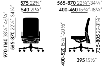
Pacific Chair avec dossier rembourré de hauteur moyenne, sans accoudoirs
