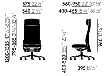
Pacific Chair avec dossier haut rembourré, sans accoudoirs
