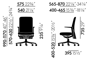
Pacific Chair avec dossier rembourré de hauteur moyenne et accoudoirs fixes
