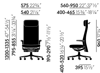
Pacific Chair avec dossier rembourré haut et accoudoirs réglables en hauteur
