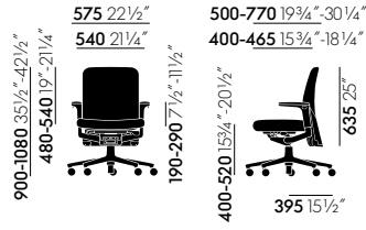
Pacific Chair avec dossier rembourré bas et accoudoirs réglables en hauteur
