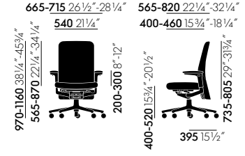
Pacific Chair avec dossier rembourré de hauteur moyenne et accoudoirs 3D
