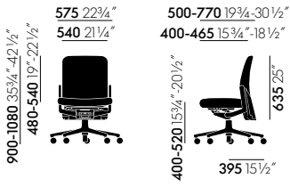
Pacific Chair avec dossier bas rembourré, sans accoudoirs
