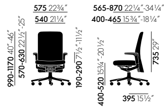
Pacific Chair avec dossier rembourré de hauteur moyenne et accoudoirs réglables en hauteur
