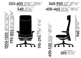
Pacific Chair avec dossier rembourré haut et accoudoirs 3D
