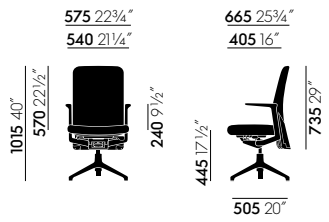
Pacific Chair avec dossier rembourré de hauteur moyenne, accoudoirs fixes et piètement à quatre branches
