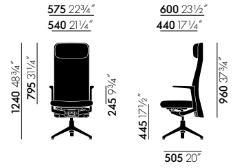
Pacific Chair avec dossier haut rembourré, accoudoirs fixes et piètement à quatre branches
