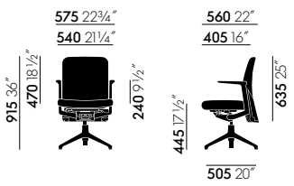
Pacific Chair avec dossier bas rembourré, accoudoirs fixes et piètement à quatre branches
